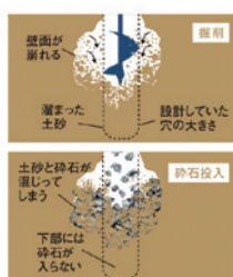
ケーシングを使用しない施工
