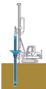
③掘削完了
